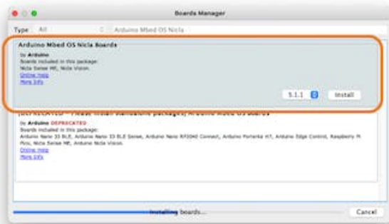
Arduino IDE 1.18
